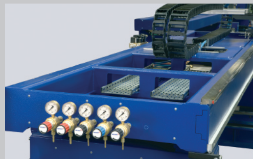
Dvojitá konstrukce mostu zaručuje vysokou tuhost při nízké hmotnosti Dvojitá konštrukcia mostu zaručuje vysokú tuhosť, pri nízkej hmotnosti
