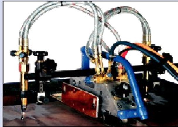
Streifenschneideeinrichtung für Streifenschnitte bis 900 mm sowie X- und Y-Fasenschnitte (Option).
